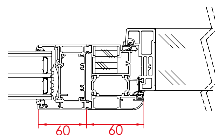
Kader + zijlicht / bovenlicht
