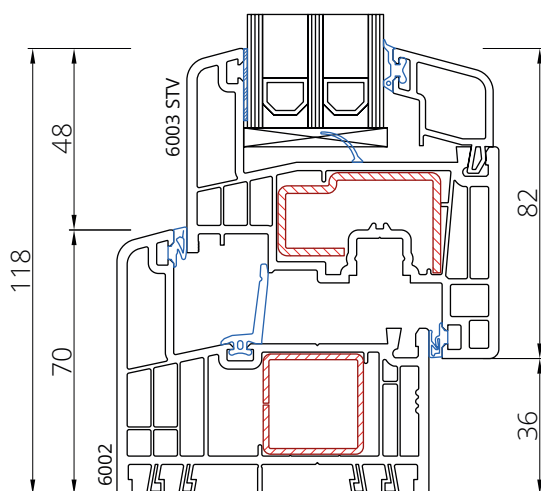
Rama 6016 Skrzydło 6003 STV
