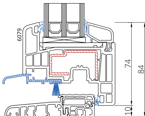
Skrzydło 6079 na progu 20 mm
