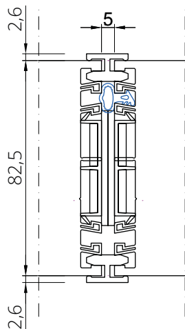
Łącznik piórkowy 3284
