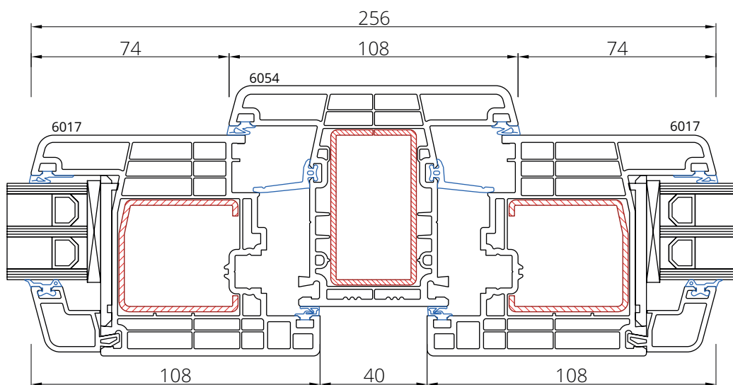
Skrzydło 6017 Słupek 6054
