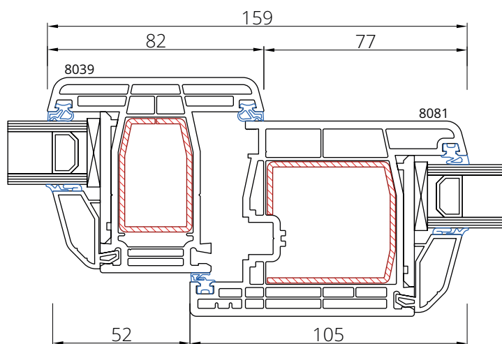
Skrzydło 8081 Słupek 8039
