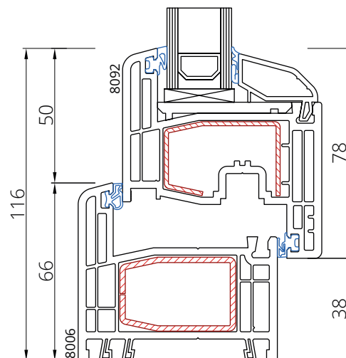
Rama 8006 Skrzydło 8092
