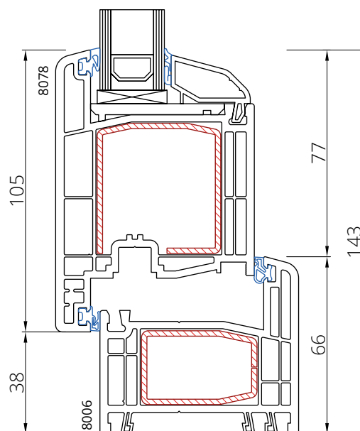
Rama 8006 Skrzydło 8078 otw. na zewnątrz
