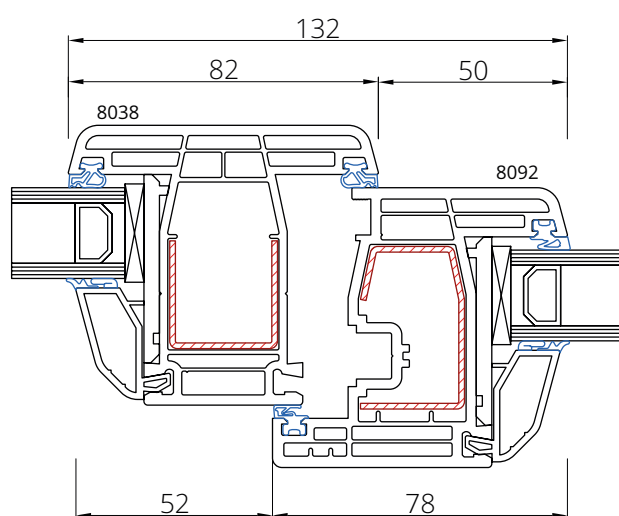
Skrzydło 8092 Słupek 8038
