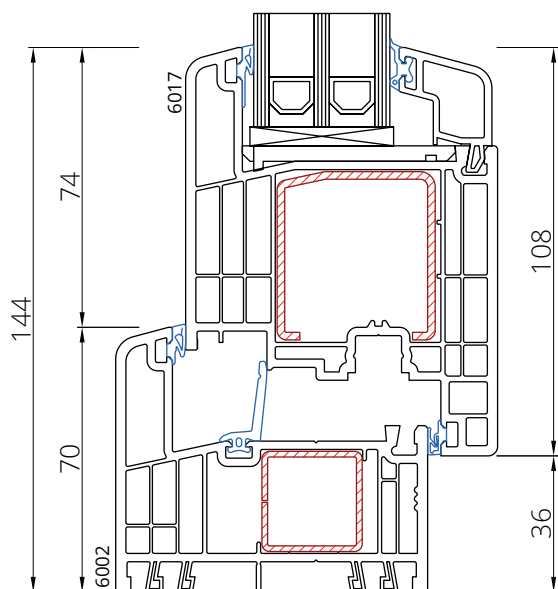
Rama 6002 Skrzydło 6017
