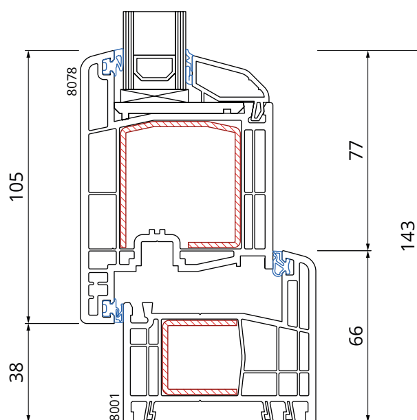
Rama 8001 Skrzydło 8078 otw. na zewnątrz
