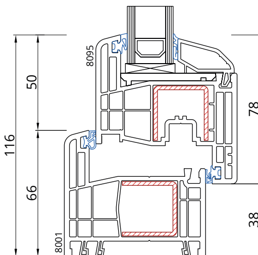
Rama 8001 Skrzydło 8095
