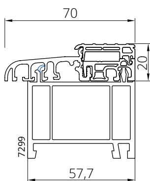
Poszerzenie gł. 57.7 GEALAN pod progiem 70mm
