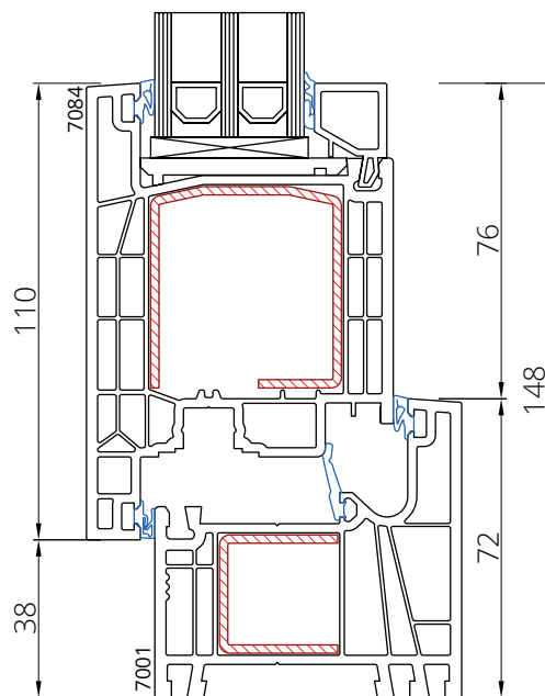
Rama 7001 Skrzydło 7084 otw. na zewnątrz
