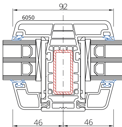
Szpros konstrukcyjny 6050
