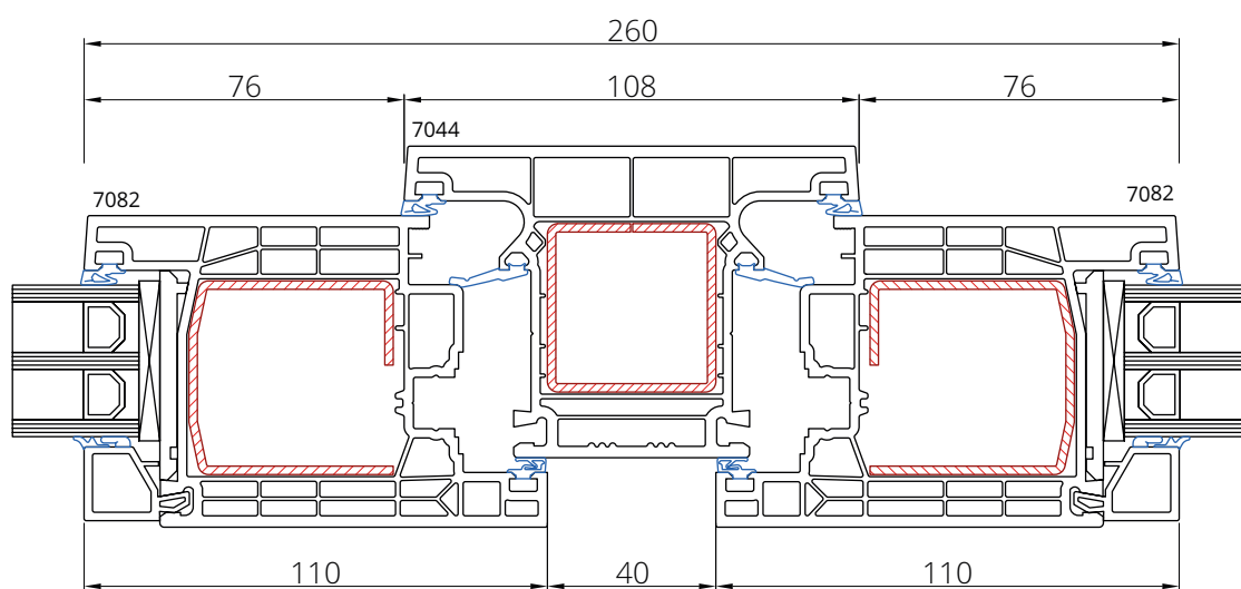
Skrzydło 7082 Słupek 7044
