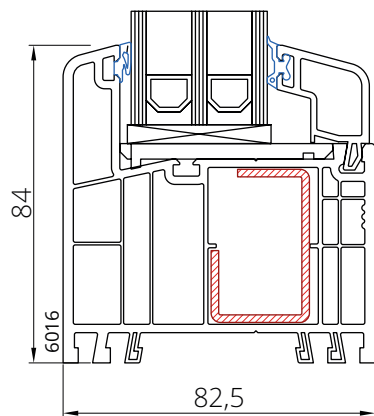
Rama 6016
