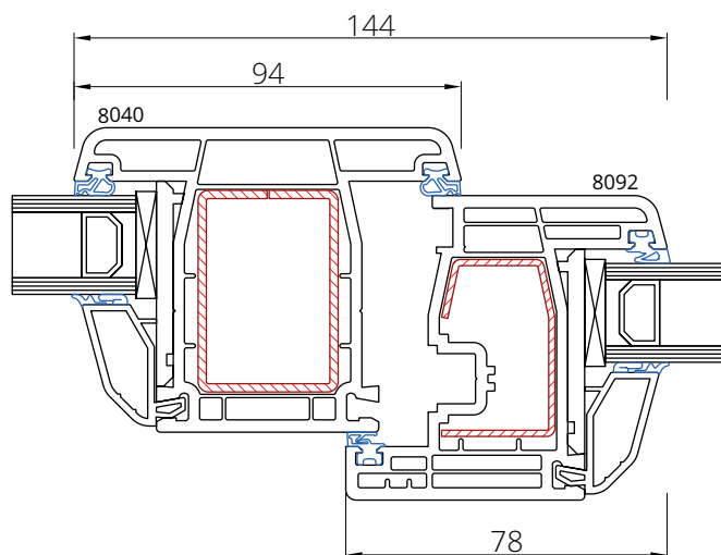
Skrzydło 8092 Słupek 8040
