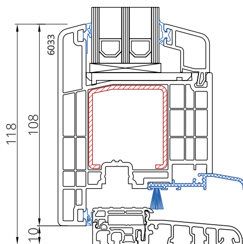
Skrzydło 6033 otw. na zewnątrz na progu 20 mm
