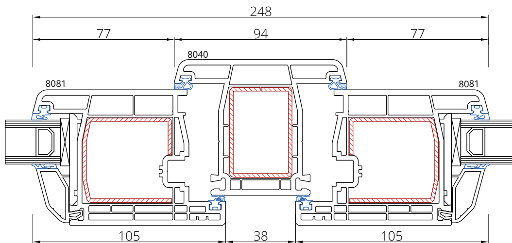
Skrzydło 8081 Słupek 8040
