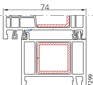
VIVA74 + profil podbalkonowy
