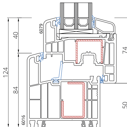
Rama 6016 Skrzydło 6079
