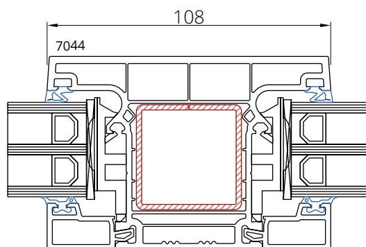
Słupek 7044
