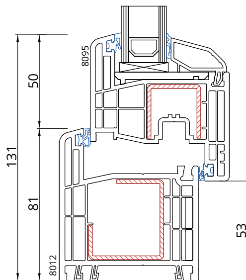
Rama 8012 Skrzydło 8095
