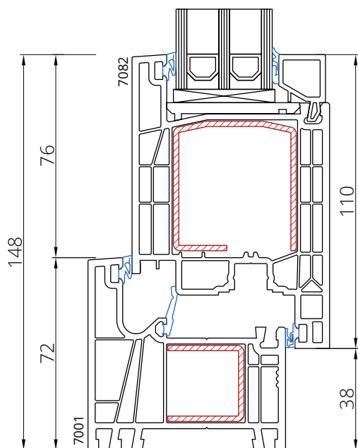
Rama 7001 Skrzydło 7082
