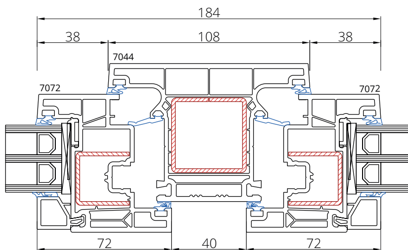
Skrzydło 7072 Słupek 7044
