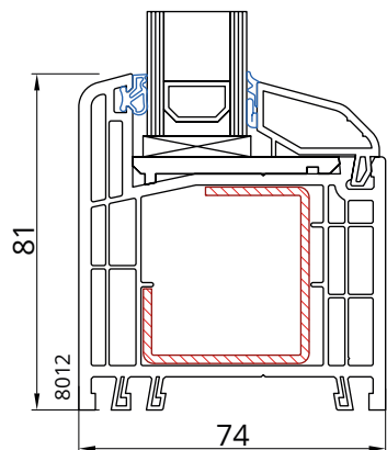
Rama 8012
