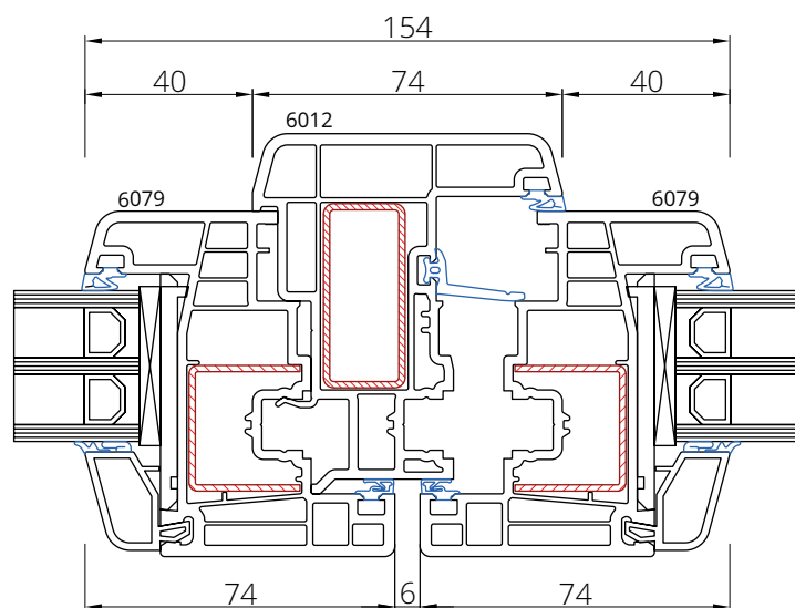
Skrzydło 6079 Słupek ruchomy 6012
