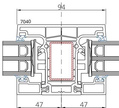
Szpros konstrukcyjny 7040
