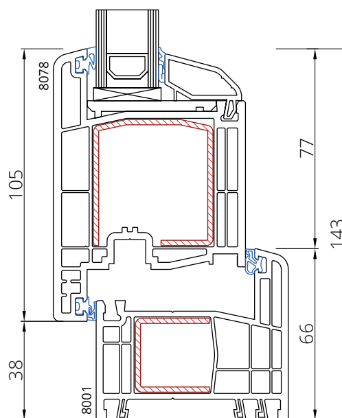
Rama 8001 Skrzydło 8078 otw. na zewnątrz
