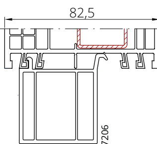
VIVA83MD + profil podbalkonowy
