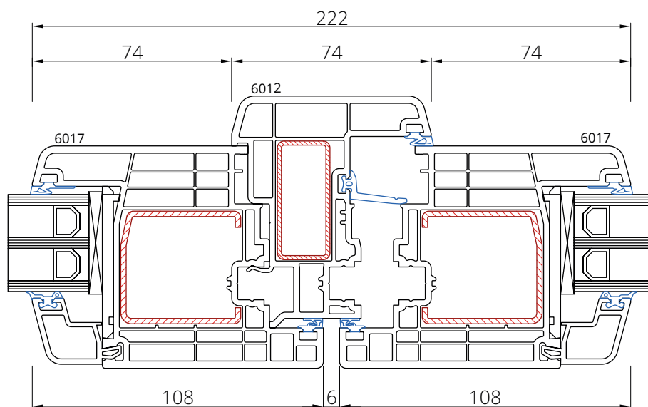
Skrzydło 6017 Słupek ruchomy 6012
