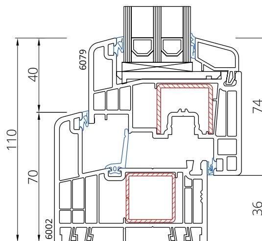
Rama 6002 Skrzydło 6079
