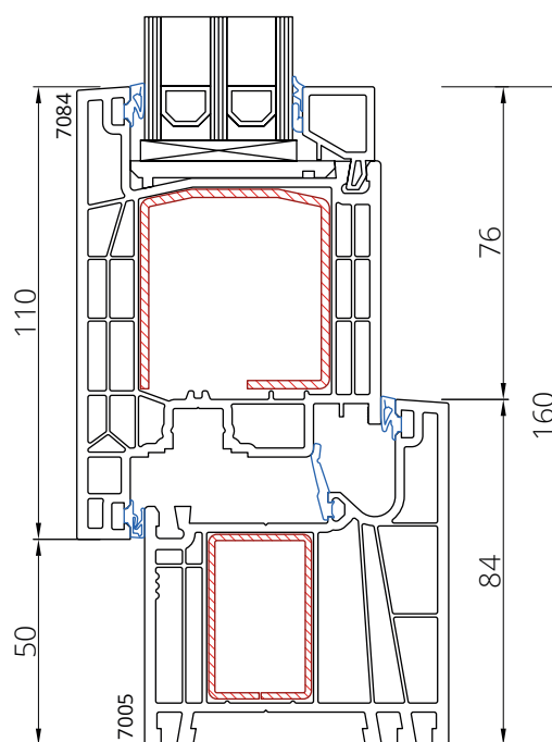
Rama 7005 Skrzydło 7084 otw. na zewnątrz
