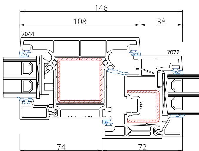
Skrzydło 7072 Słupek 7044
