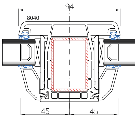
Szpros konstrukcyjny 8040
