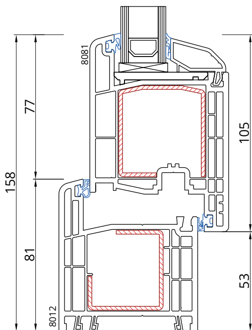
Rama 8012 Skrzydło 8081
