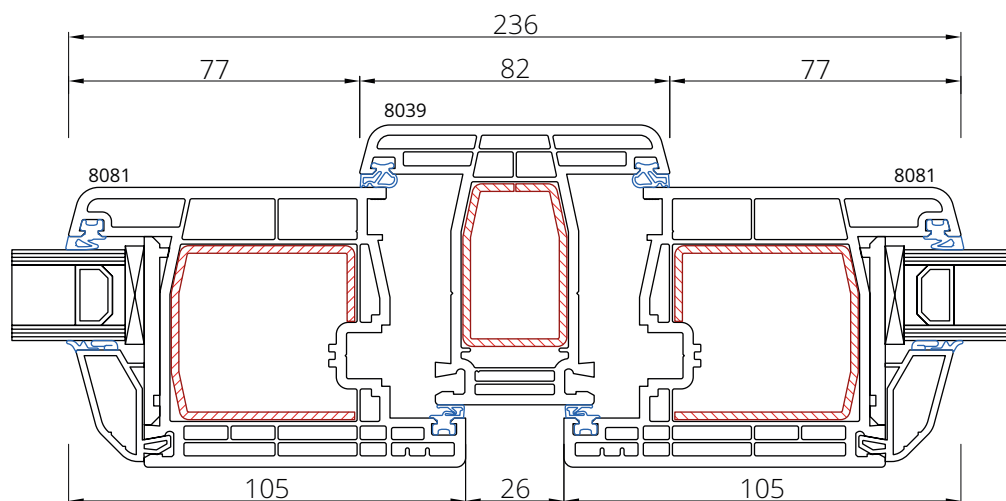
Skrzydło 8081 Słupek 8039
