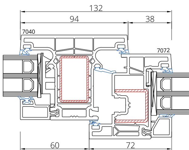
Skrzydło 7072 Słupek 7040
