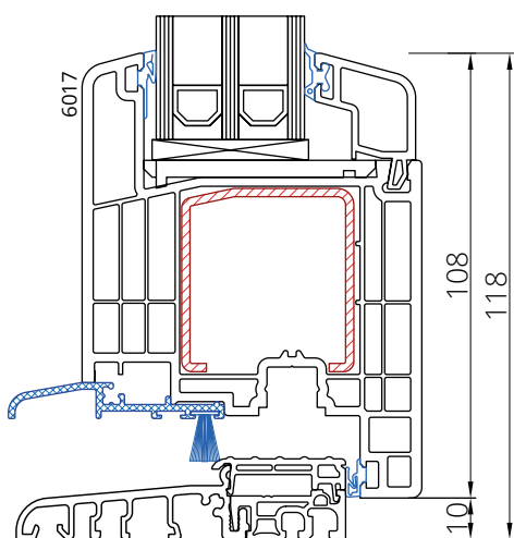
Skrzydło 6017 na progu 20 mm
