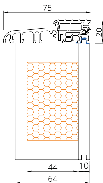
IHPV pod progiem 75mm
