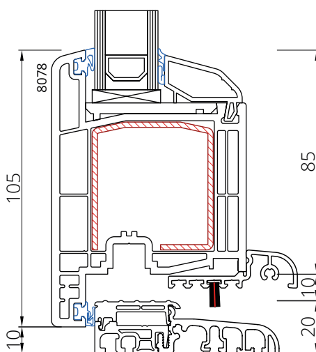
Skrzydło 8078 otw. na zewnątrz na progu 20 mm
