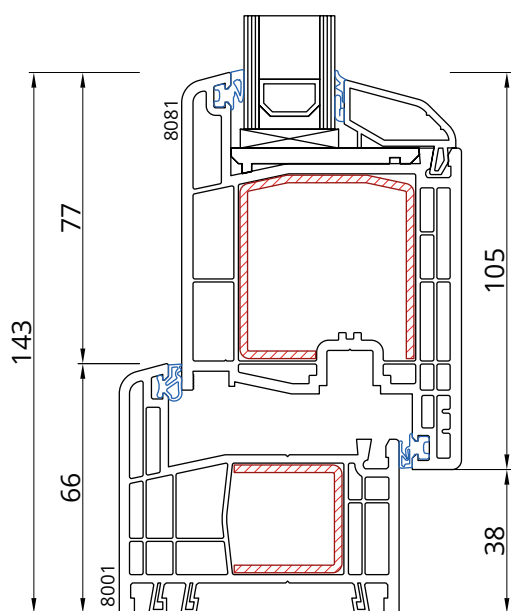
Rama 8001 Skrzydło 8081
