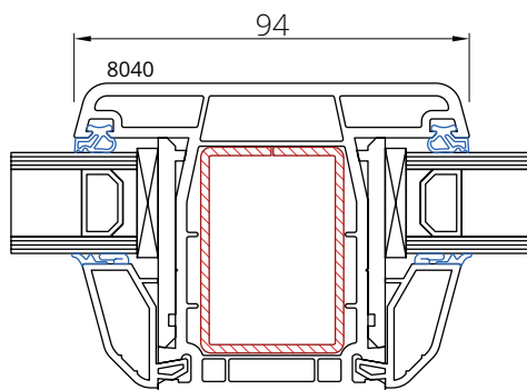
Słupek 8040
