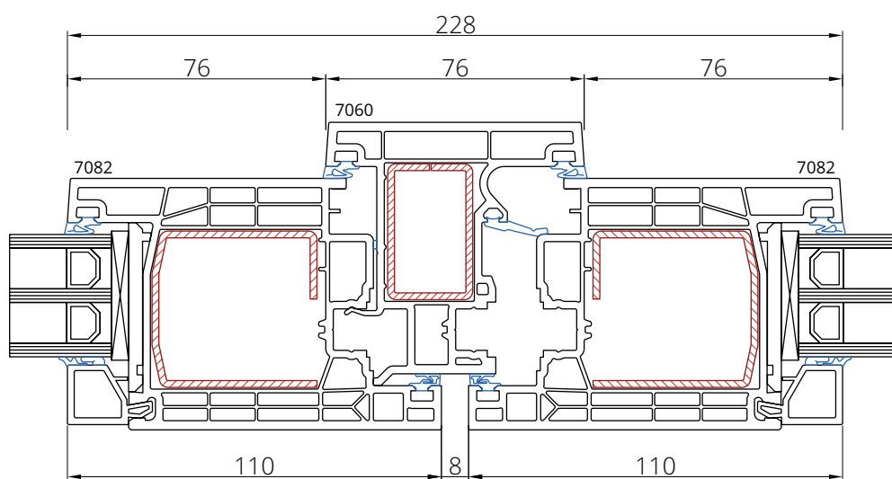
Skrzydło 7082 Słupek ruchomy 7060
