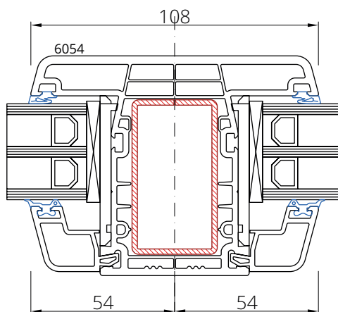
Szpros konstrukcyjny 6054
