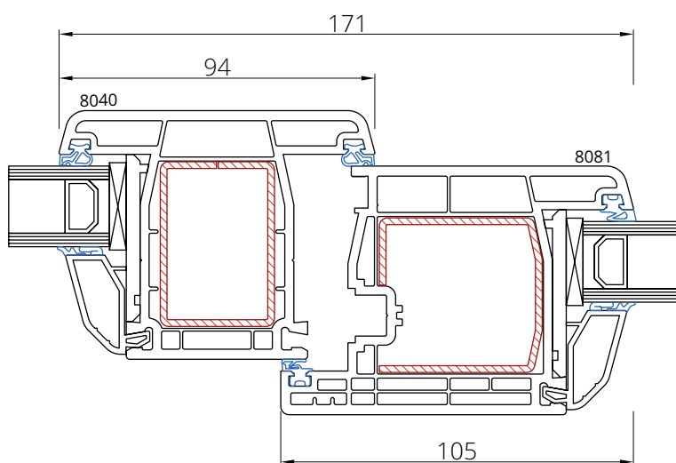
Skrzydło 8081 Słupek 8040
