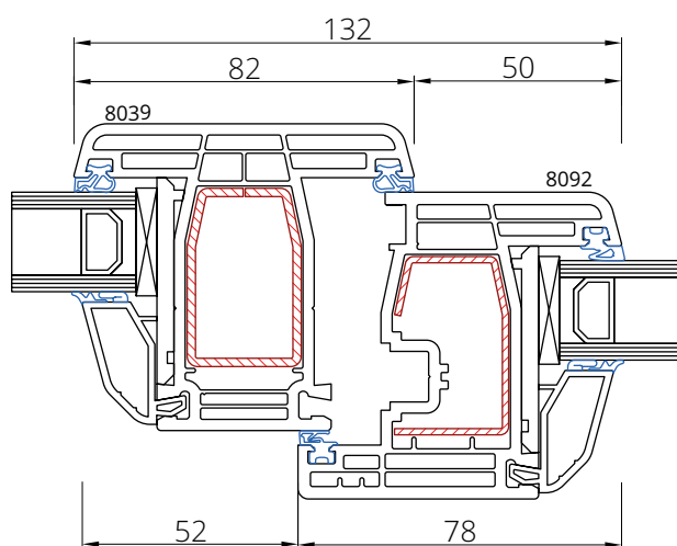
Skrzydło 8092 Słupek 8039
