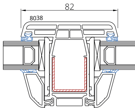
Słupek 8038
