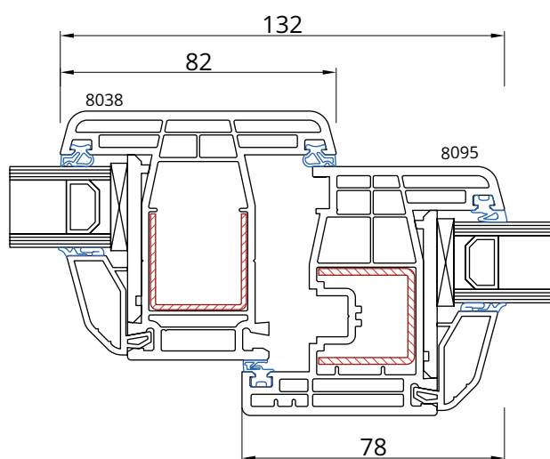
Słupek 8038 Skrzydło 8095
