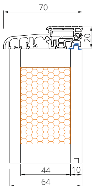
IHPV pod progiem 70mm
