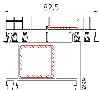
VIVA83MD + profil podbalkonowy
