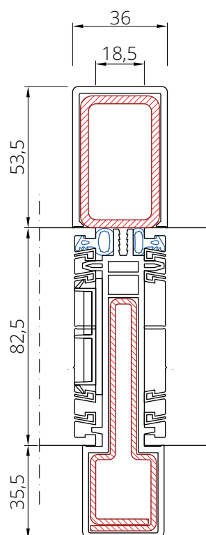
Łącznik 5204 zarga 2249
