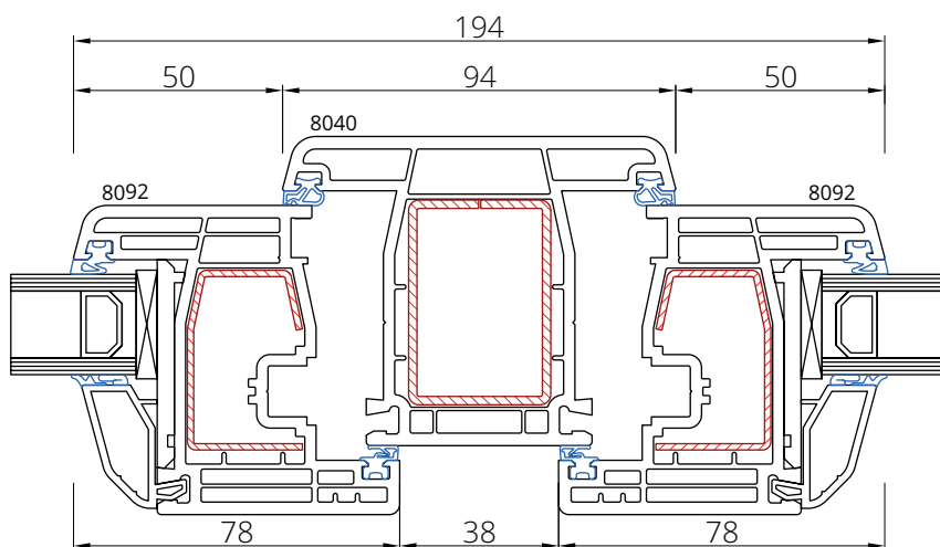
Skrzydło 8092 Słupek 8040
