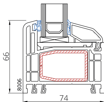
Rama 8006
