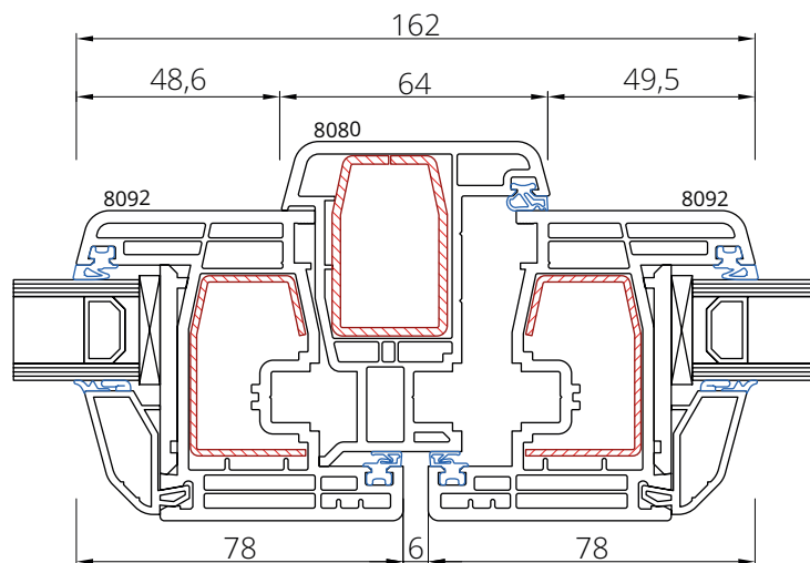
Skrzydło 8092 Słupek ruchomy 8080
