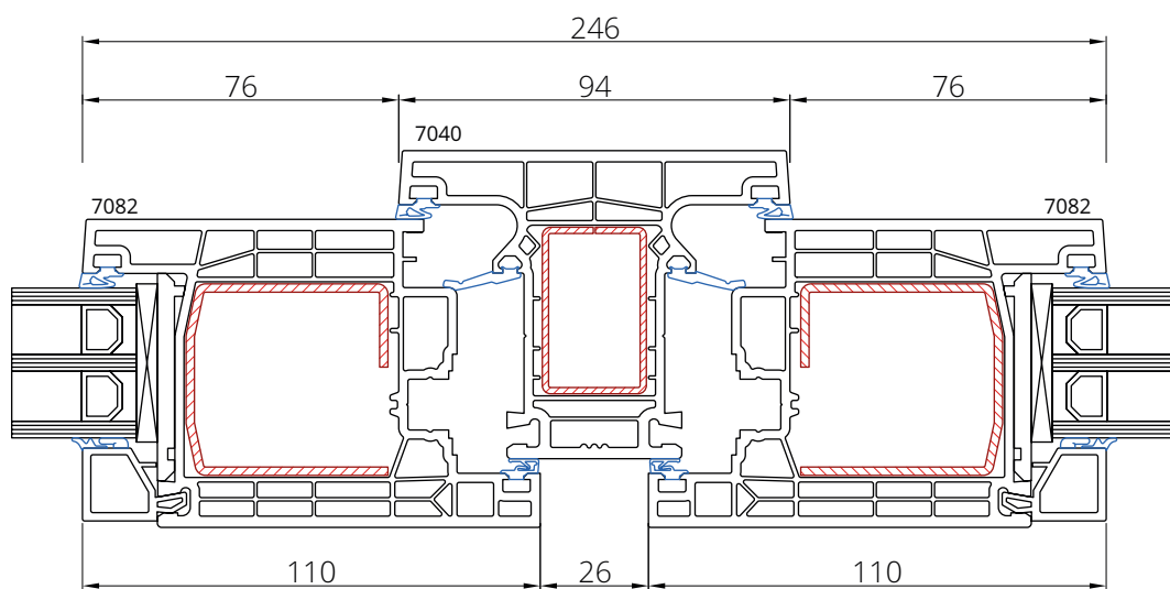
Skrzydło 7082 Słupek 7040
