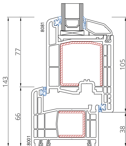
Rama 8001 Skrzydło 8081
