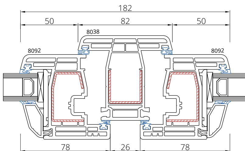
Skrzydło 8092 Słupek 8038
