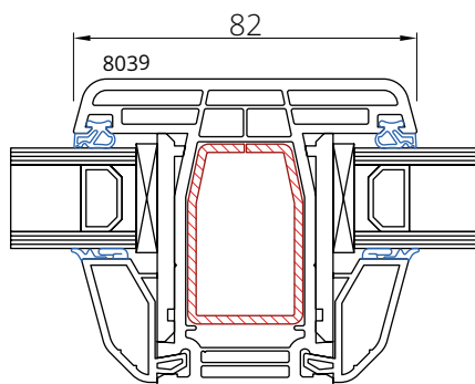
Słupek 8039
