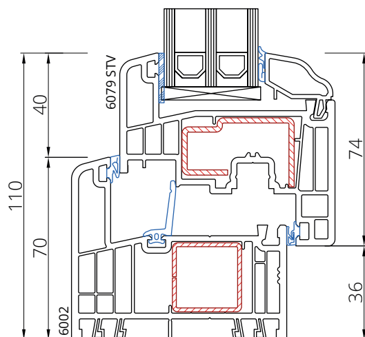
Rama 6016 Skrzydło 6079 STV
