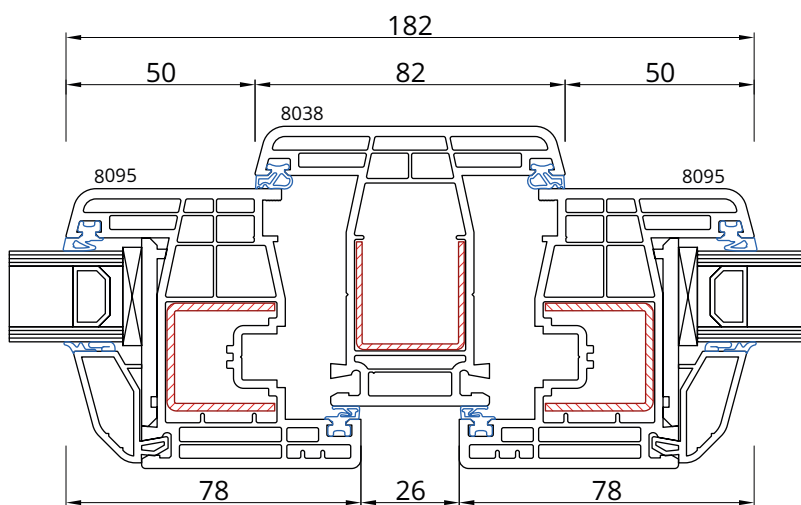
Słupek 8038 Skrzydło 8095
