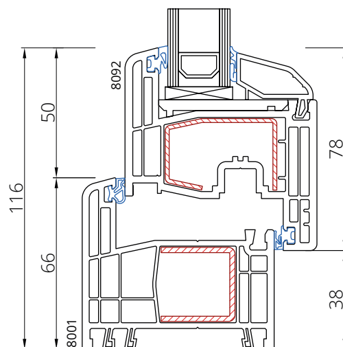
Rama 8001 Skrzydło 8092
