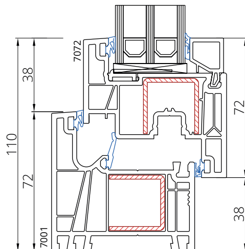
Rama 7001 Skrzydło 7072
