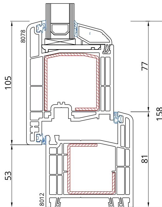
Rama 8012 Skrzydło 8078 otw. na zewnątrz
