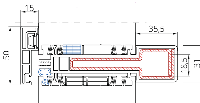
Łącznik 5204 okapnik 3245
