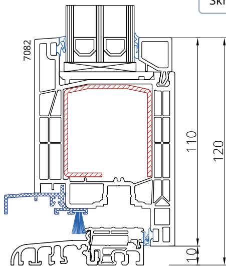
Skrzydło 7082 na progu 20 mm
