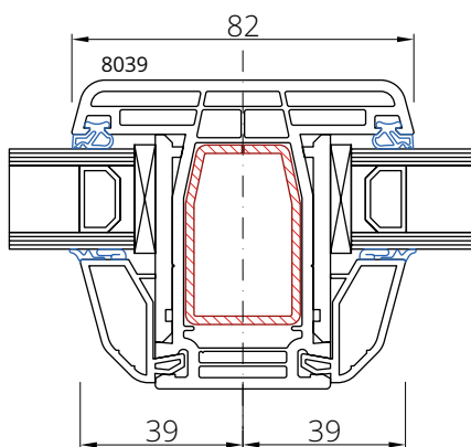
Szpros konstrukcyjny 8039
