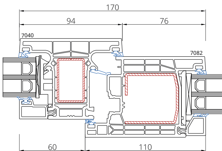
Skrzydło 7082 Słupek 7040
