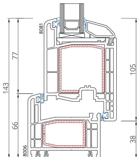
Rama 8006 Skrzydło 8081
