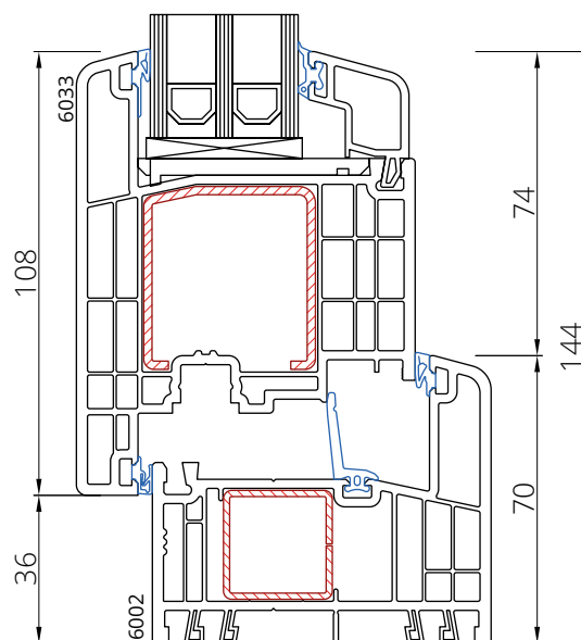
Rama 6002 Skrzydło 6033 otw. na zewnątrz
