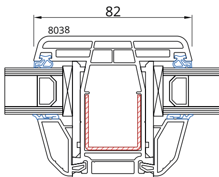
Słupek 8038
