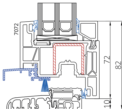
Skrzydło 7072 na progu 20 mm
