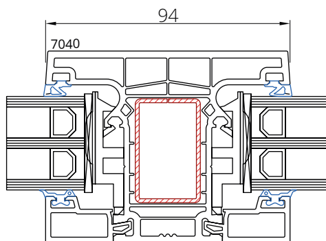
Słupek 7040
