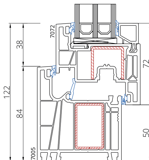
Rama 7005 Skrzydło 7072
