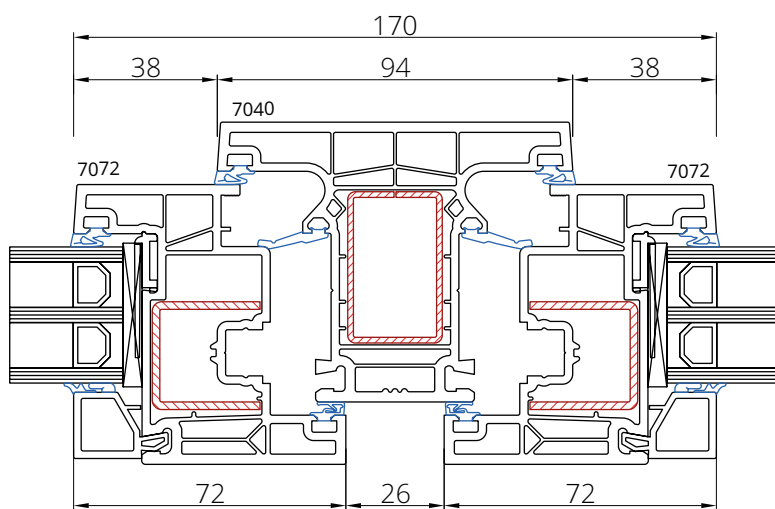
Skrzydło 7072 Słupek 7040
