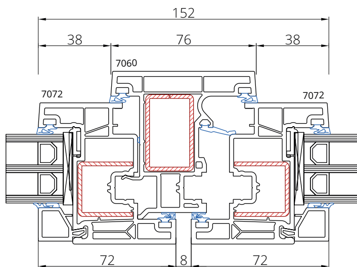
Skrzydło 7072 Słupek ruchomy 7060
