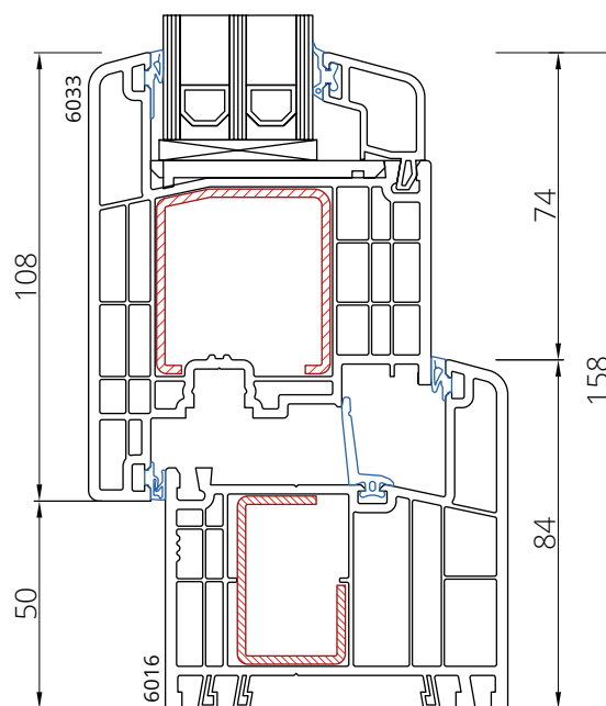
Rama 6016 Skrzydło 6033 otw. na zewnątrz
