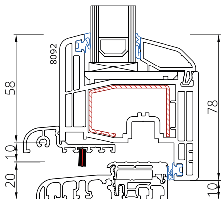
Skrzydło 8092 na progu 20 mm
