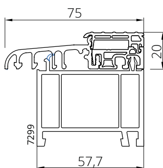
Poszerzenie gł. 57.7 GEALAN pod progiem 75mm
