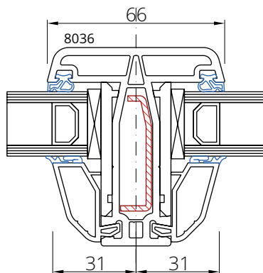
Szpros konstrukcyjny 8036
