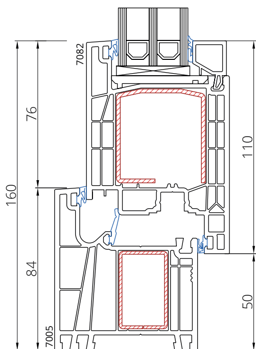
Rama 7005 Skrzydło 7082
