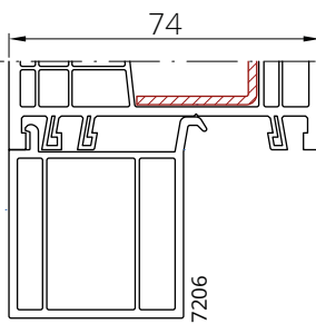
VIVA74 + profil podbalkonowy
