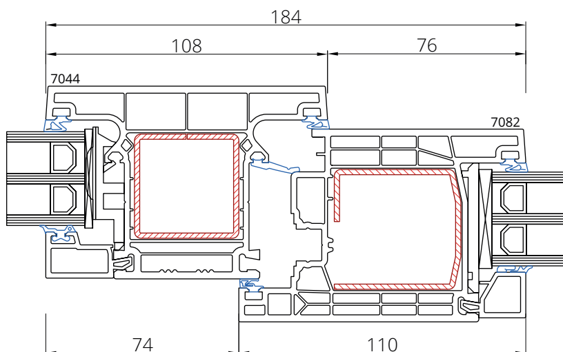
Skrzydło 7082 Słupek 7044
