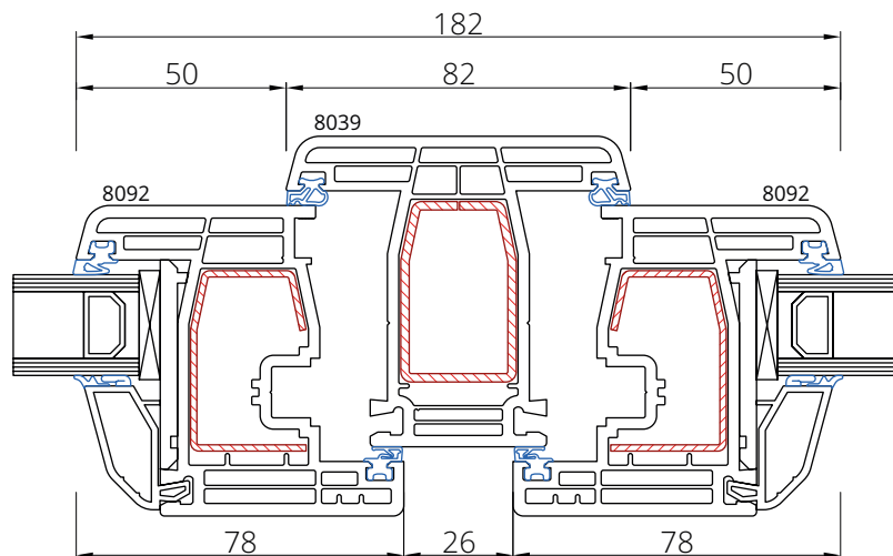
Skrzydło 8092 Słupek 8039
