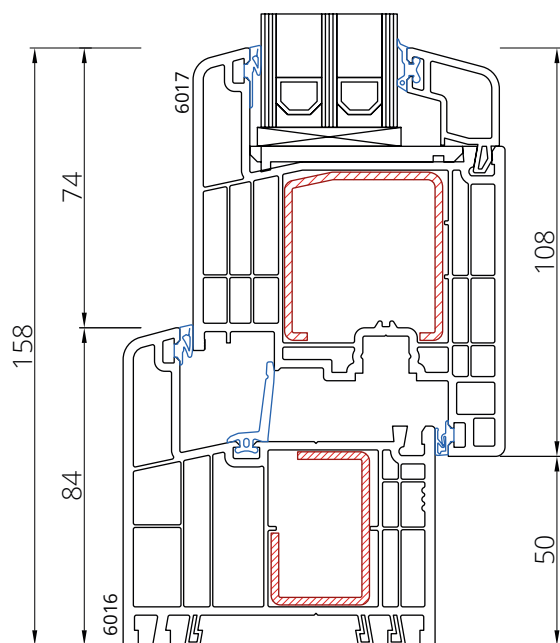
Rama 6016 Skrzydło 6017
