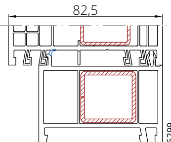
VIVA83MD + profil podbalkonowy
