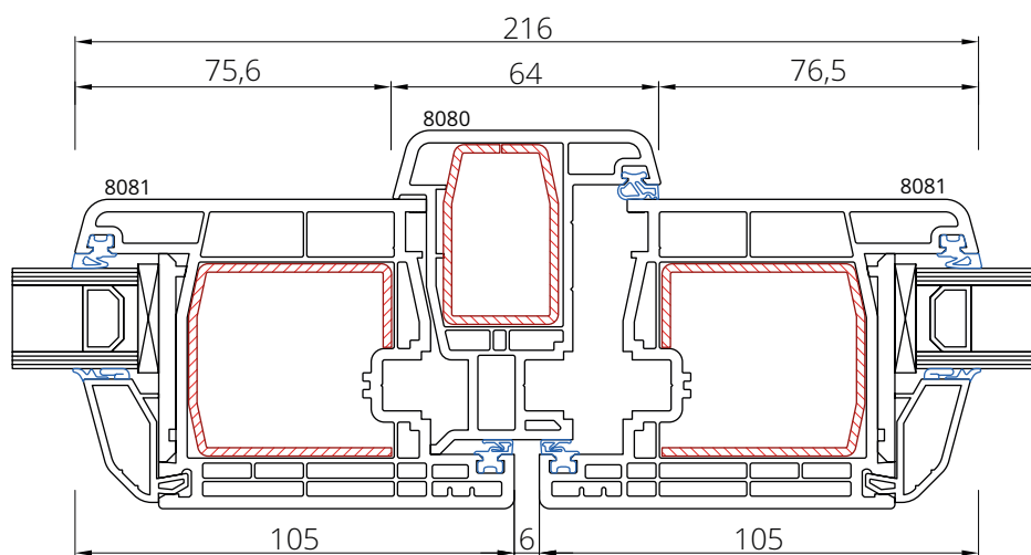
Skrzydło 8081 Słupek ruchomy 8080
