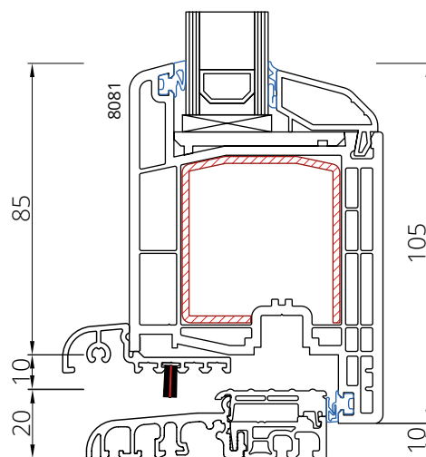
Skrzydło 8081 na progu 20 mm
