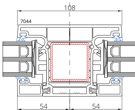
Szpros konstrukcyjny 7044
