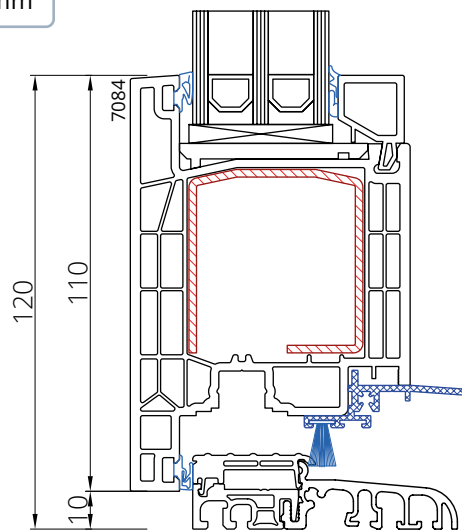
Skrzydło 7084 otw. na zewnątrz na progu 20 mm
