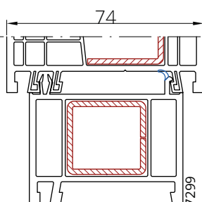
VIVA74 + profil podbalkonowy
