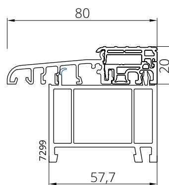
Poszerzenie gł. 57.7 GEALAN pod progiem 80mm
