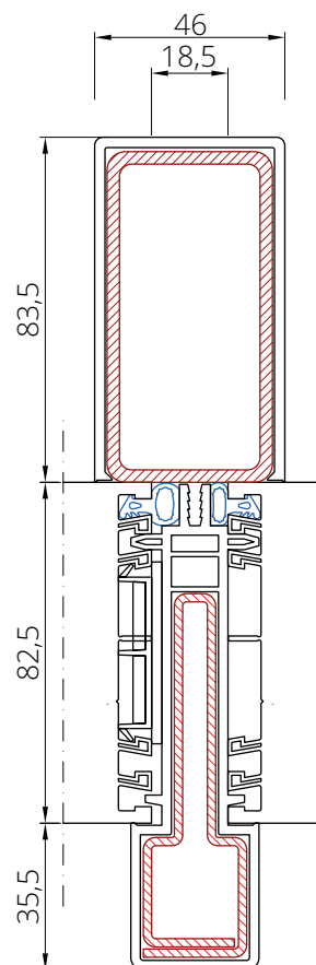
Łącznik 5204 zarga 3240
